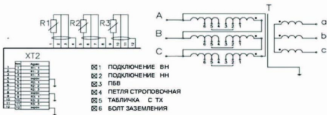
Схема электрическая принципиальная трансформатор ТС3
